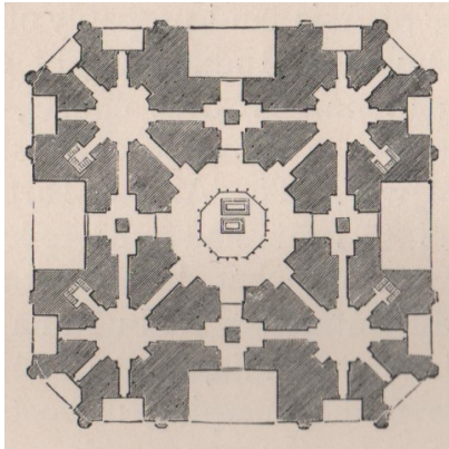
Grundriss Kuppelbau Tj, Indien
